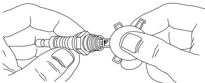
Рис. 4-5. Измерение зазора свечи зажигания
